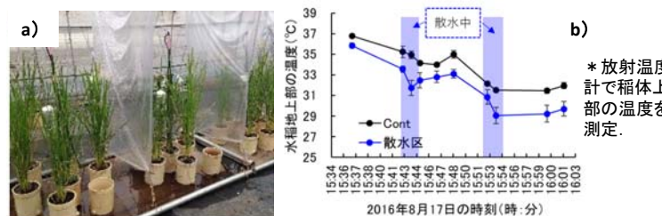
図2 スプリンクラーによる稲体周囲への散水実験
